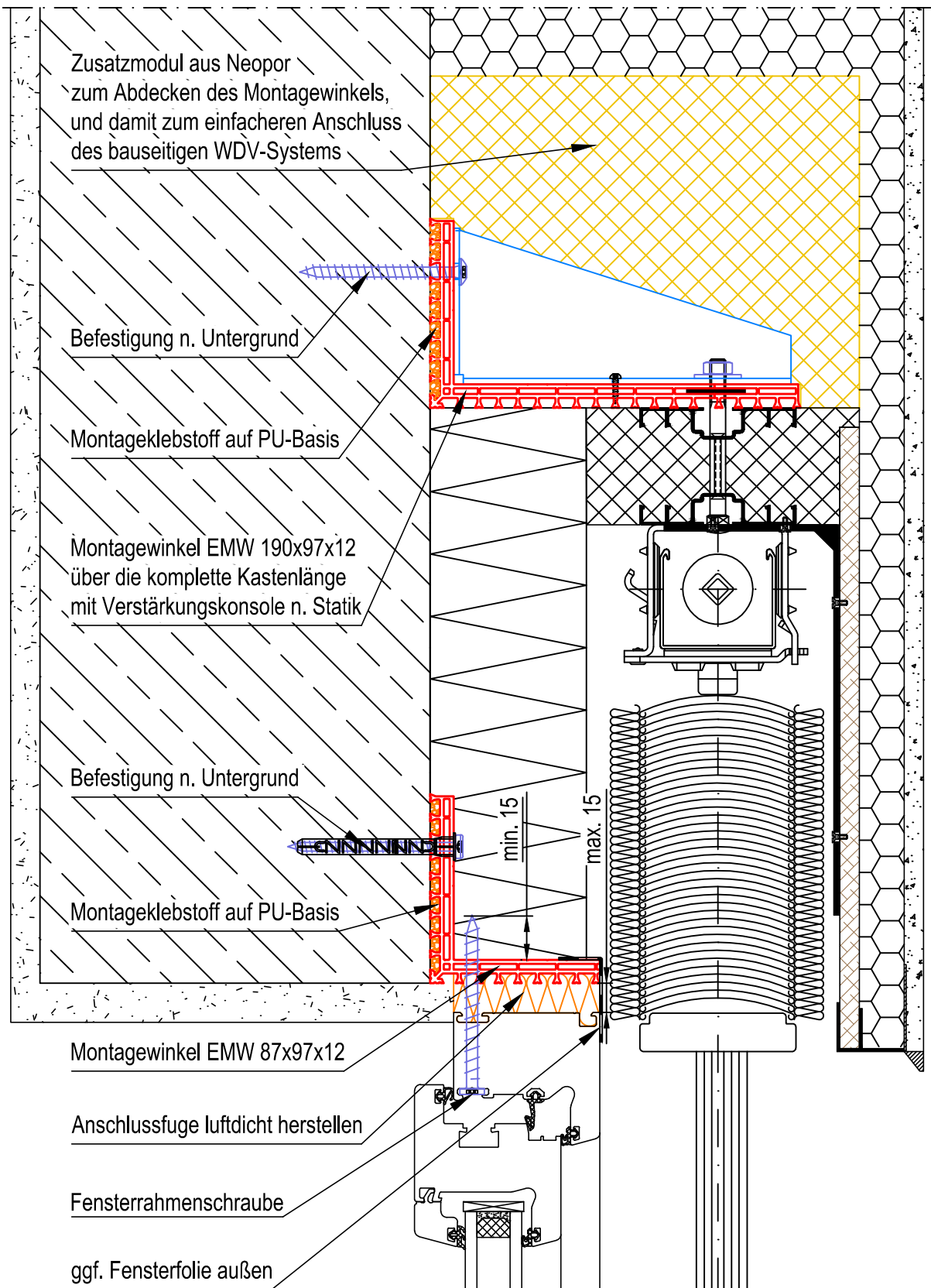
Schnitt C-C
