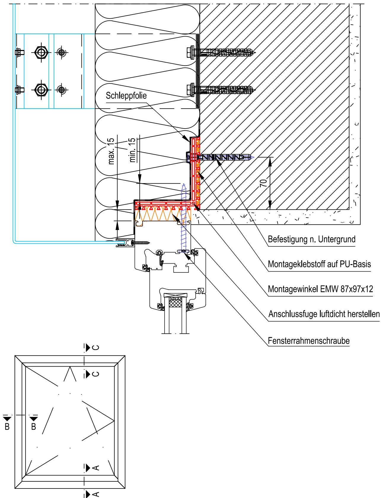
Schnitt C-C
