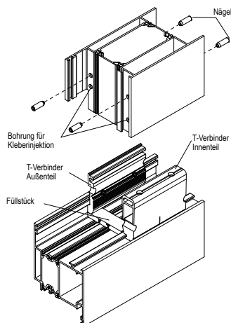
T-Verbinder Set (n)
