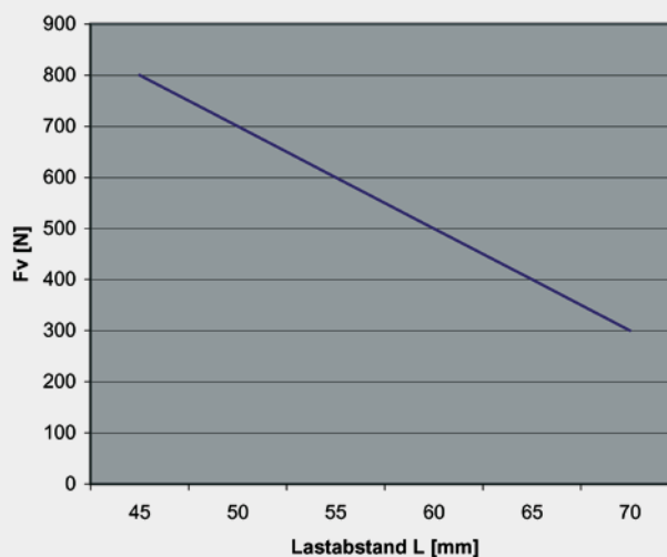
Maximale Vertikalkraft Richtwerte auf Basis System Schüco
