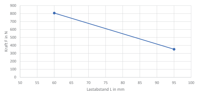
Richtwerte für Lastrichtung Querkraft im eingebauten Zustand bei einer max. Verformung von 8 mm
